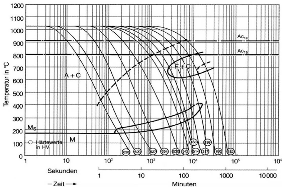
ZTU-Schaubild (kontinuierlich)
